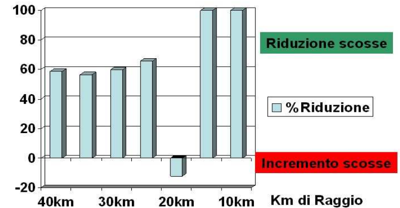
Valvola Antisismica su S.Pietro in Casale analisi su 26 anni
